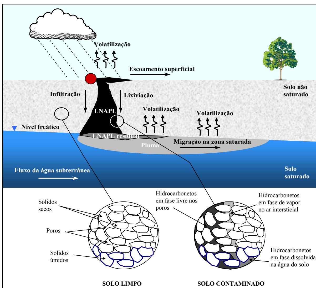
FIGURA 2.3 – Representação esquemática de um derramamento de hidrocarbonetos do petróleo e a migração dos contaminantes no aquífero.
