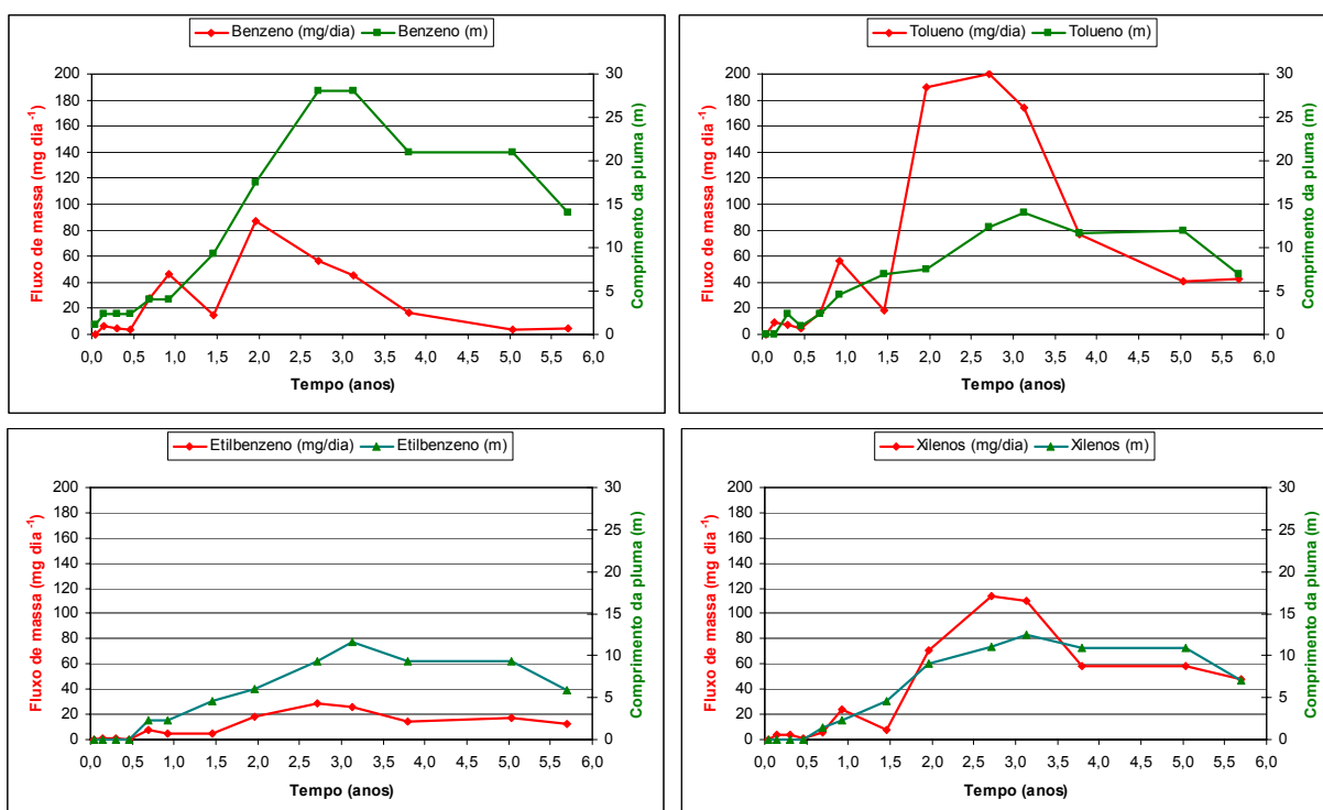
FIGURA 4.19 – Variação temporal do fluxo de massa de compostos BTEX e do comprimento das plumas de contaminação.
