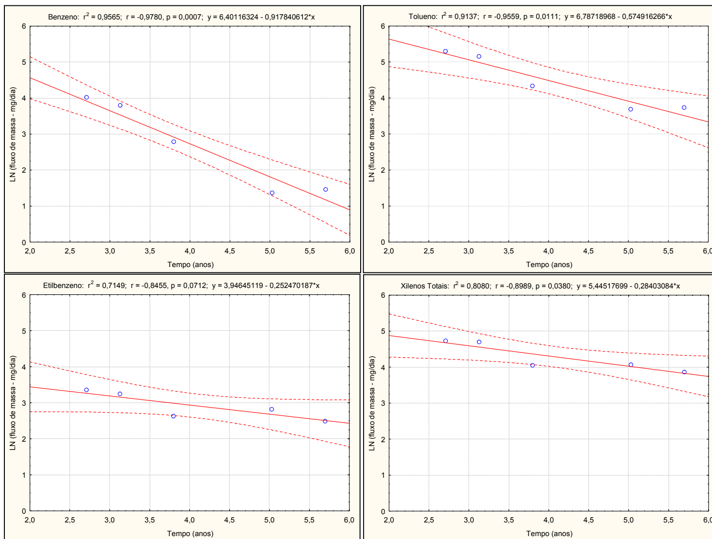
FIGURA 4.10 – Ajuste do Modelo de Caixa aos dados de fluxo de massa dos compostos BTEX após o etanol ter sido exaurido da fonte de contaminação, no período de 2,0 a 5,7 anos. A linha central representa a função ajustada e as linhas externas tracejadas definem a faixa de predição do modelo com 95% de confiança.
