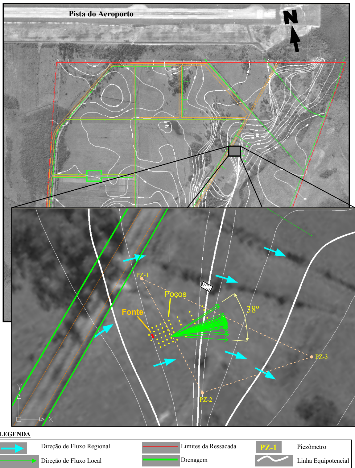
FIGURA 3.3 - Variações na direção do fluxo da água subterrânea no período de junho/1998 a outubro/1999.
