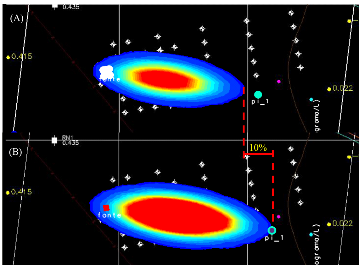
FIGURA 4.23 – Resultados da simulação do comprimento da pluma de benzeno sem etanol (A) e com etanol (B) com o modelo SCBR. A diferença entre o comprimento da pluma A e da pluma B foi de 10%.
