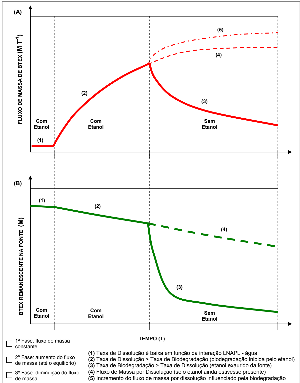
FIGURA 4.16 - Modelo conceitual da variação do fluxo de massa (A) e da intemperização (B) dos hidrocarbonetos do petróleo influenciado pela presença do etanol na fonte de contaminação. Modelo válido para derramamentos de gasolina comercial brasileira (24% de etanol) em pulso.
