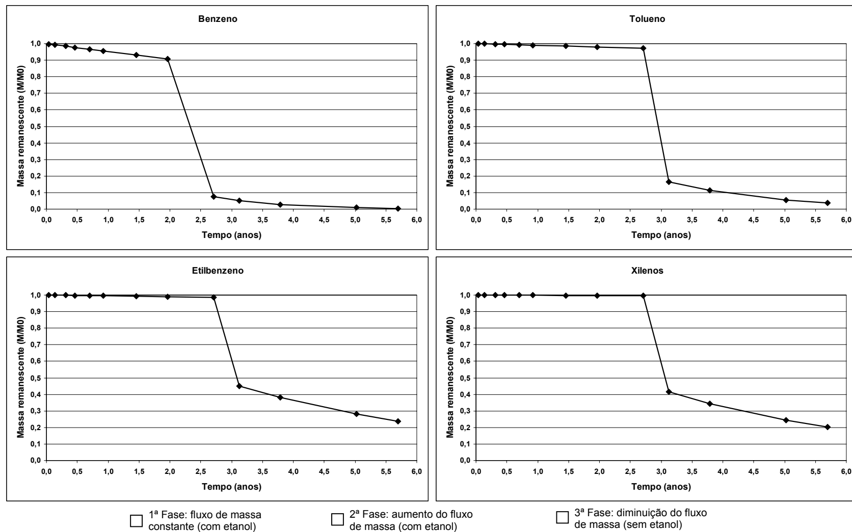
FIGURA 4.13 – Gráficos da intemperização dos compostos BTEX presentes na fonte de contaminação a partir de um derramamento controlado de 100 L de gasolina (24% etanol). Em 5,7 anos após o derramamento, a massa intemperizada de benzeno, tolueno, etilbenzeno e xilenos da fonte foi de 99, 97, 76 e 80% respectivamente.
