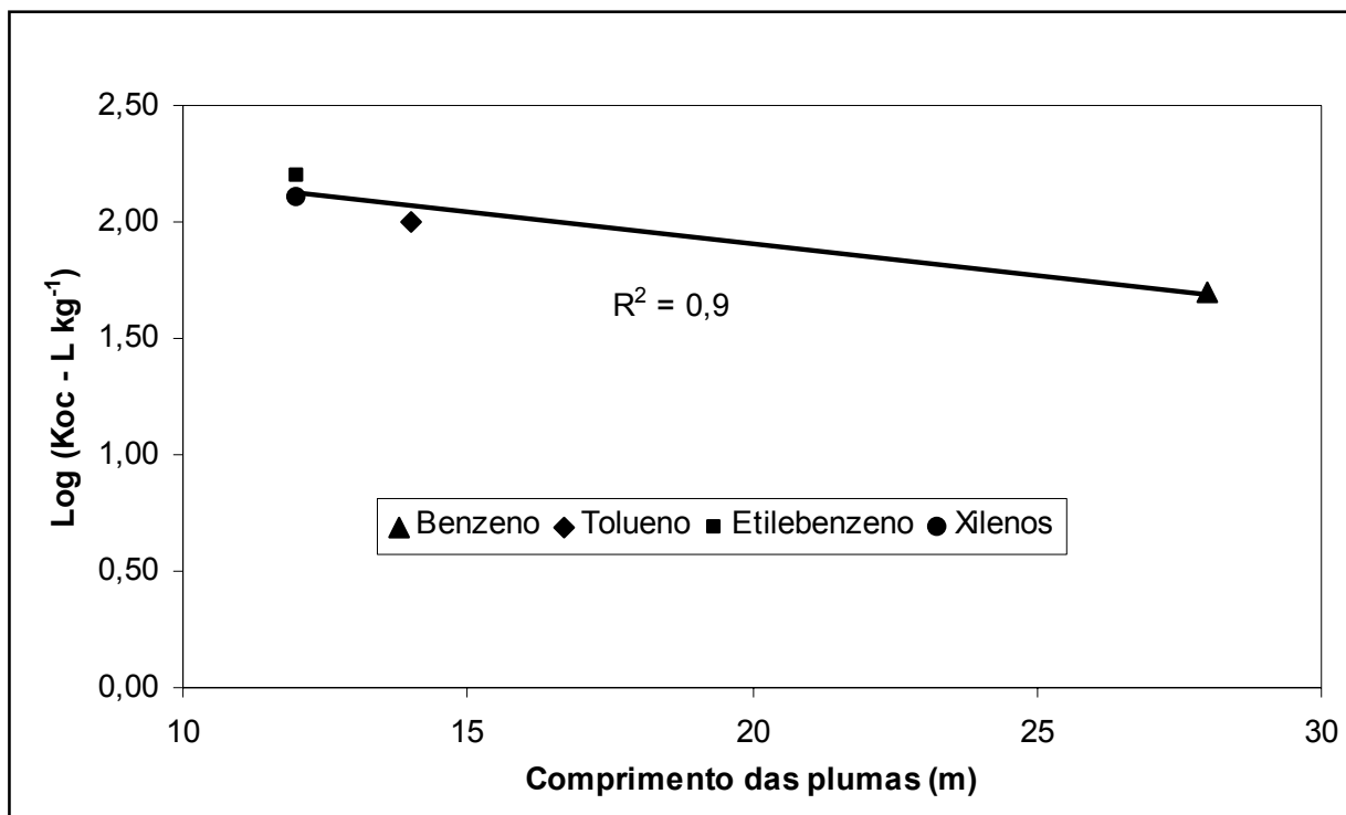
FIGURA 4.21 – Associação entre o coeficiente de sorção ( K_{oc} ) dos compostos BTEX e o comprimento das plumas.
