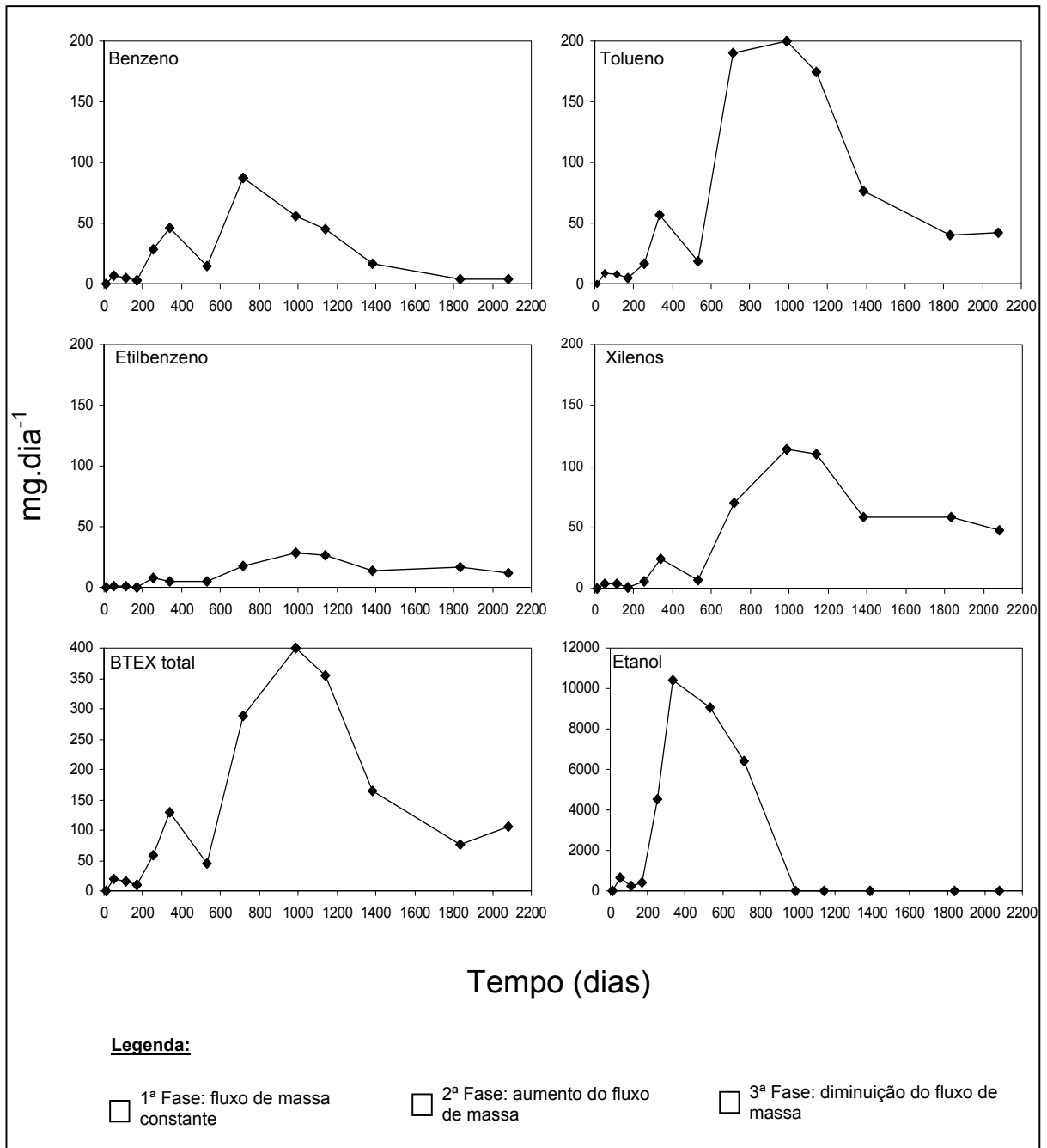
FIGURA 4.1 – Fluxo de massa de compostos BTEX e etanol na região da fonte. Obs.: A brusca diminuição no fluxo de massa para os compostos BTEX na 7ª coleta (531 dias) não pode ser explicada com as informações disponíveis.
