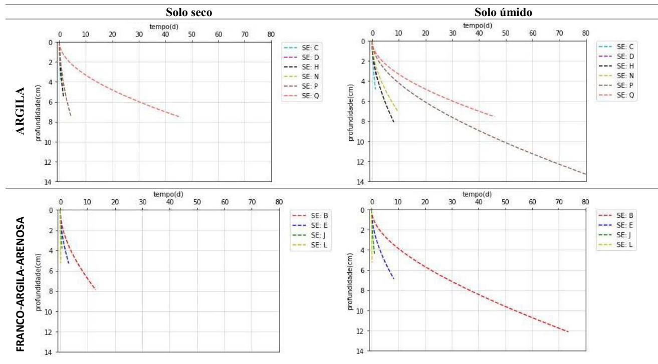
Figura 5.18. Resultados das simulações das frentes de migração obtidos por meio do algoritmo.
