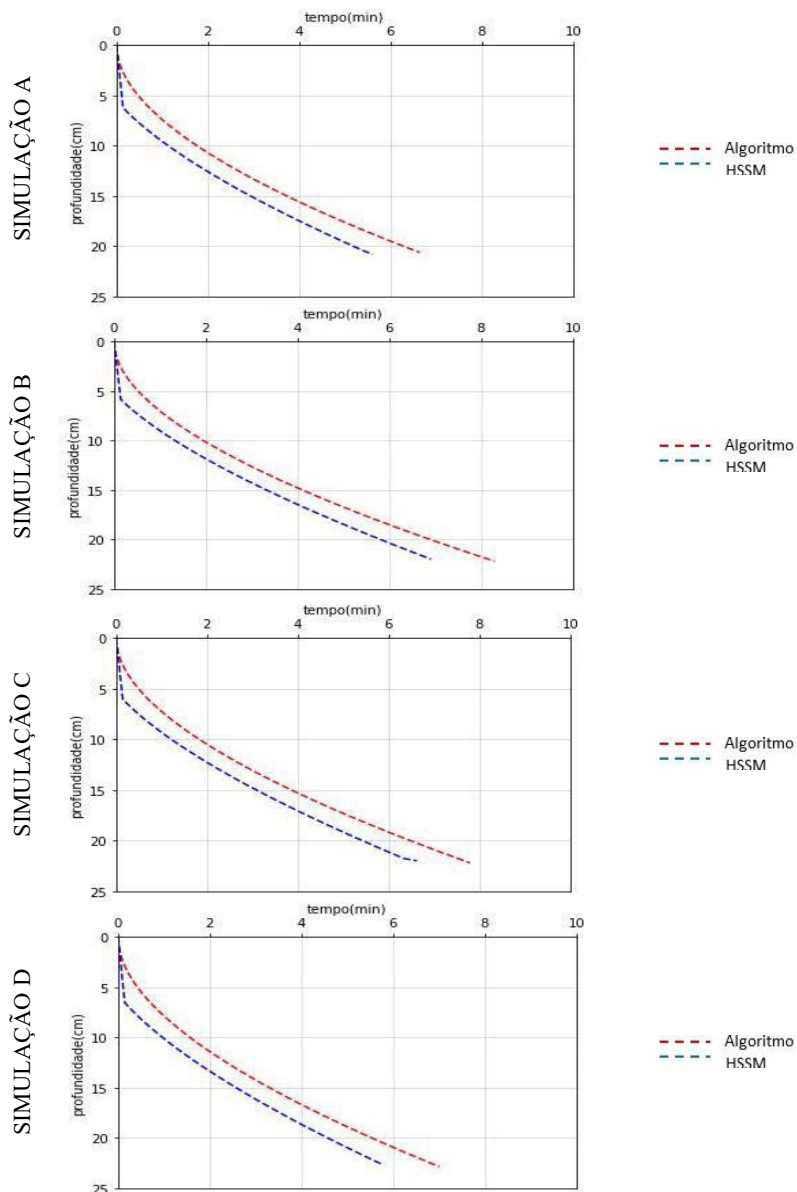
Figura 5.2. Resultados da frente de migração das simulações (A, B, C e D) para o cenário I.
