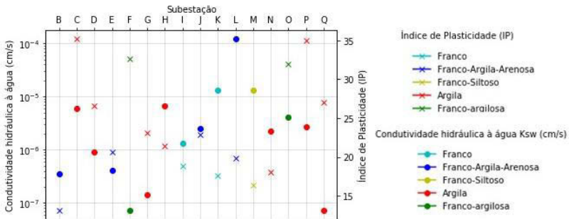
Figura 5.9. Resultados das análises do índice de plasticidade e da condutividade hidráulica por subestação de energia elétrica
