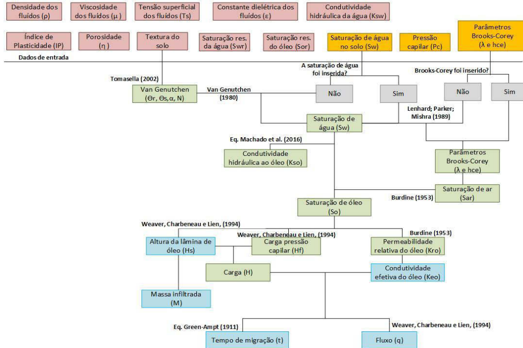
Figura 4.3. Fluxograma da metodologia aplicada para a determinação da frente de escoamento. Legenda: Rosa-dados obrigatório; Laranja – dados opcionais; Verde – Parâmetros intermediários; Azul -Parâmetros finais.
