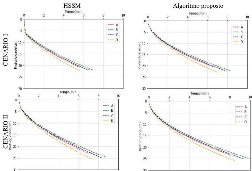
Figura 5.5. Comparação entre os resultados das frentes de migração obtidos pelo HSSM e pelo Algoritmo proposto.
