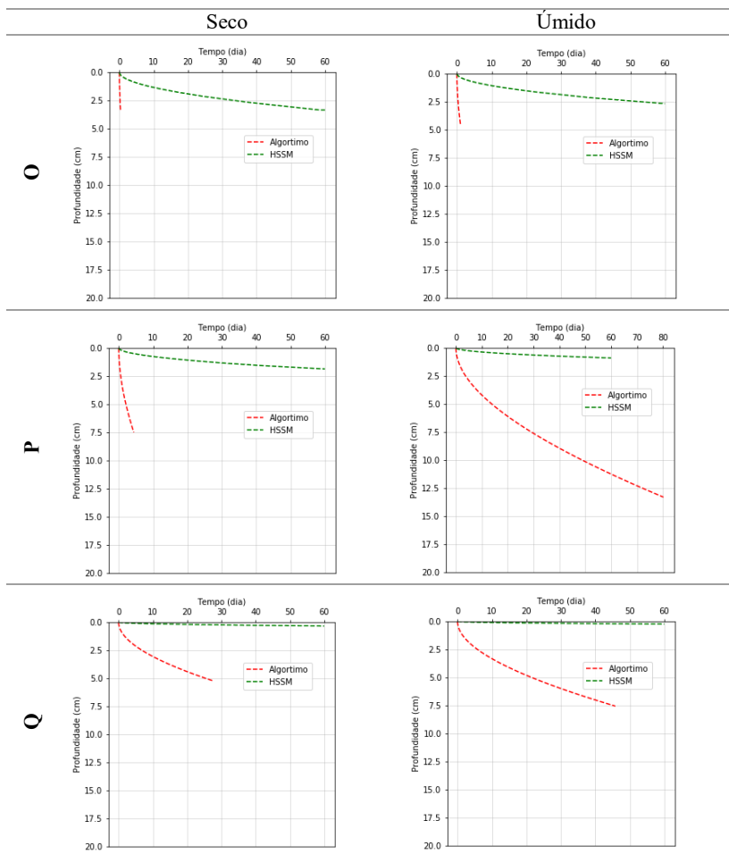
Figura 5.16. Comparação entre as frentes de migrações do óleo mineral isolante obtido por meio do HSSM (verde) e do algoritmo (vermelho) (CONTINUAÇÃO).
