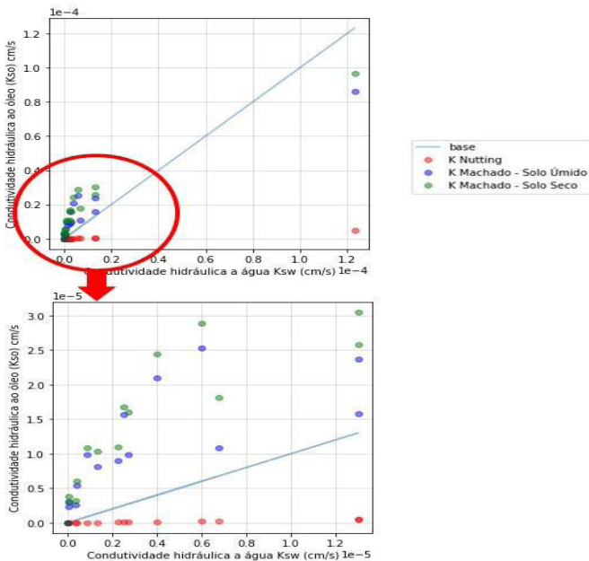
Figura 5.12. Comparação entre os valores da condutividade hidráulica ao óleo obtida pela equação de Machado et al. (2016) e pela equação de Nutting (1934) com a condutividade hidráulica à água
