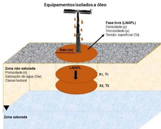
Figura 4.2. Modelo esquemático do escoamento do LNAPL em zona não saturada.
