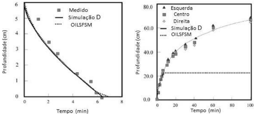
Figura 3.12. Verificação da equação de Green-Ampt (1911) utilizada no OILSFSM. a) Altura da lâmina de óleo b) Infiltração.
