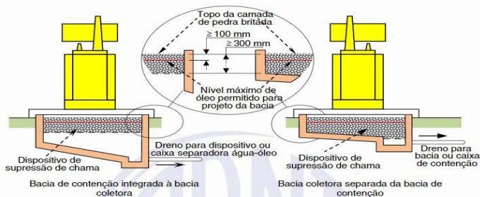
Figura 3.4. Sistema de proteção contra incêndio (bacias coletoras).
