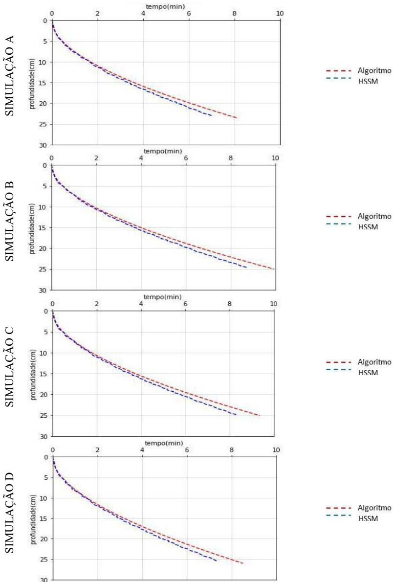
Figura 5.3. Resultados da frente de migração das simulações (A, B, C e D) para o cenário II.
