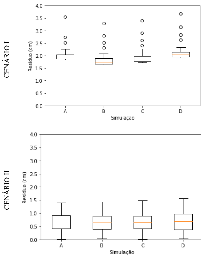
Figura 5.4. Box Plot dos resíduos entre os resultados do HSSM e do algoritmo proposto.
