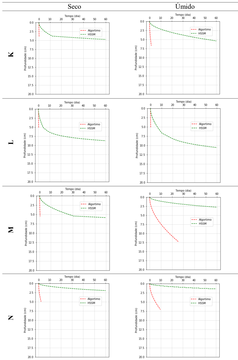
Figura 5.15. Comparação entre as frentes de migrações do óleo mineral isolante obtido por meio do HSSM (verde) e do algoritmo (vermelho) (CONTINUAÇÃO).
