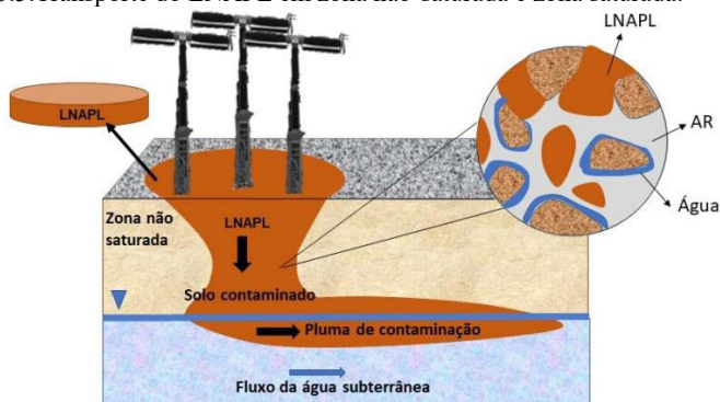
Figura 3.5. Transporte do LNAPL em zona não-saturada e zona saturada.
