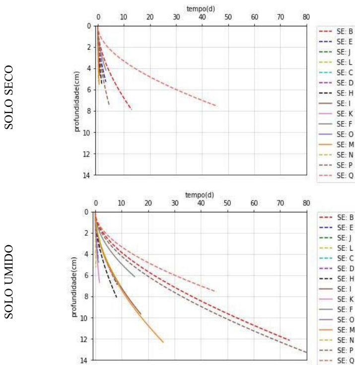
Figura 5.17. Resultado das simulações, utilizando o algoritmo, para as subestações de acordo com a saturação de água no solo.
