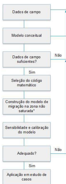
Figura 4.1. Fluxograma para o desenvolvimento do algoritmo de migração de LNAPL na zona não saturada.
