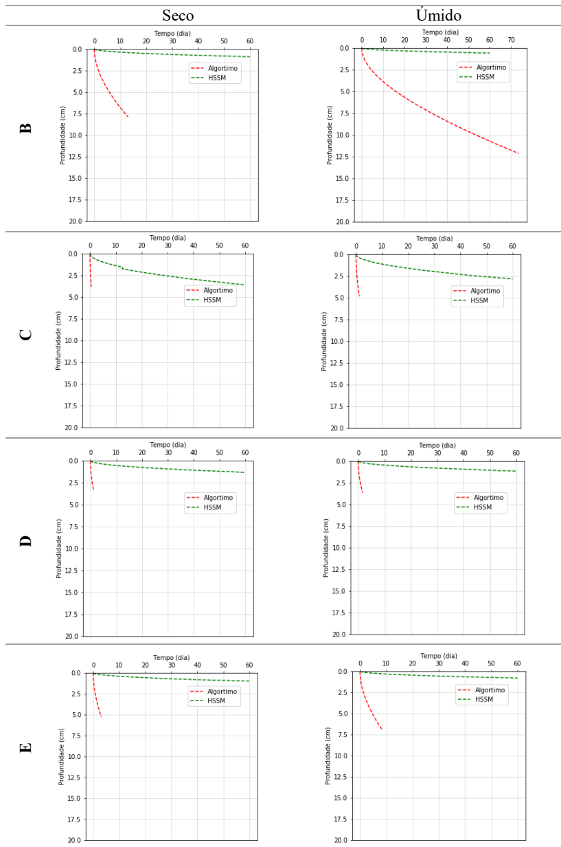
Figura 5.13. Comparação entre as frentes de migrações do óleo mineral isolante obtido por meio do HSSM (verde) e do algoritmo (vermelho) (CONTINUAÇÃO).
