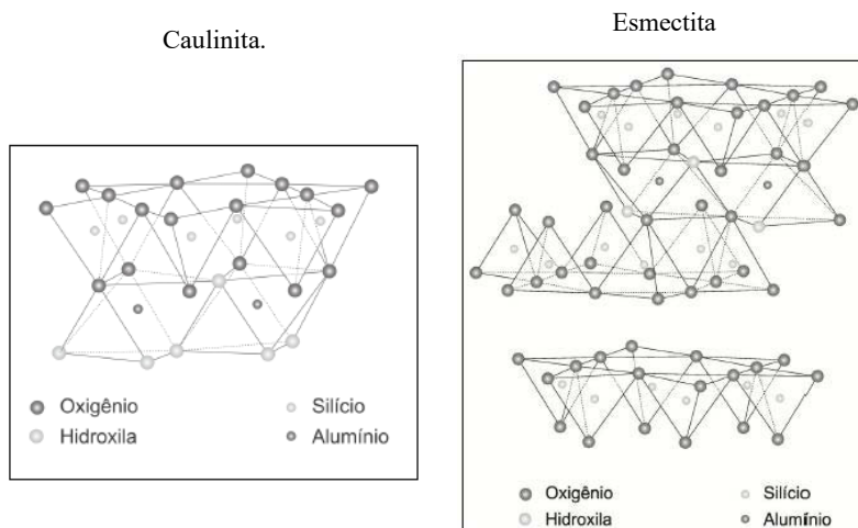
Figura 3.9. Estrutura dos argilominerais filossilicatos bilaminares e trilaminares.
