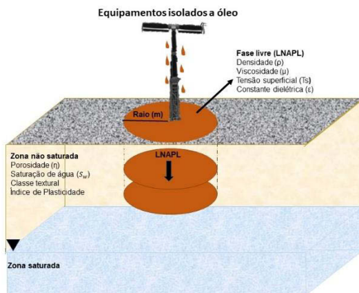
Figura 5.1. Modelo conceitual utilizado para a construção do algoritmo.
