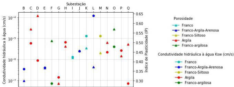
Figura 5.10. Resultados das análises da porosidade e da condutividade hidráulica por subestação de energia elétrica
