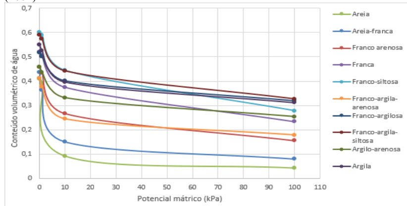
Figura 3.10. Curva de retenção obtida a partir dos dados de Hodnett e Tomasella, (2002).
