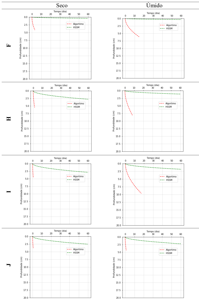
Figura 5.14. Comparação entre as frentes de migrações do óleo mineral isolante obtido por meio do HSSM (verde) e do algoritmo (vermelho) (CONTINUAÇÃO).
